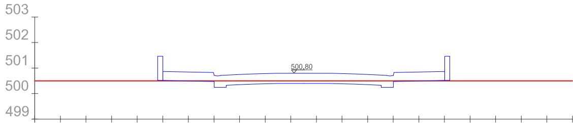
SECCION TRANSVERSAL 6
