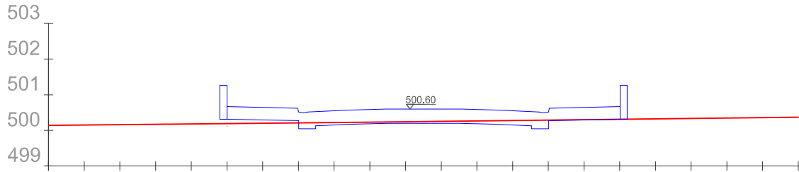
SECCION TRANSVERSAL 5
