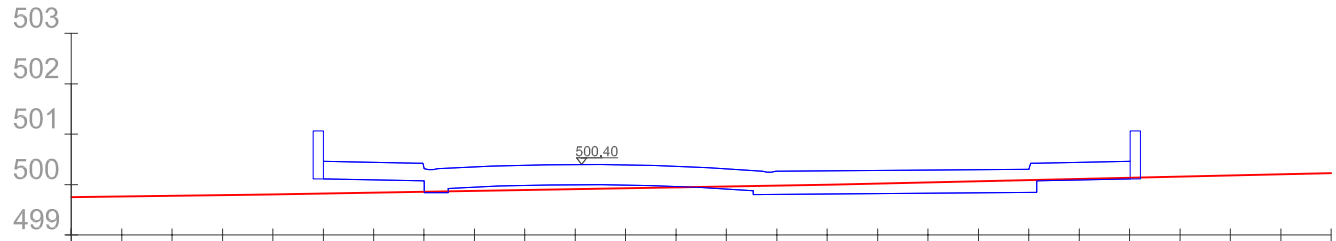
SECCION TRANSVERSAL 3
