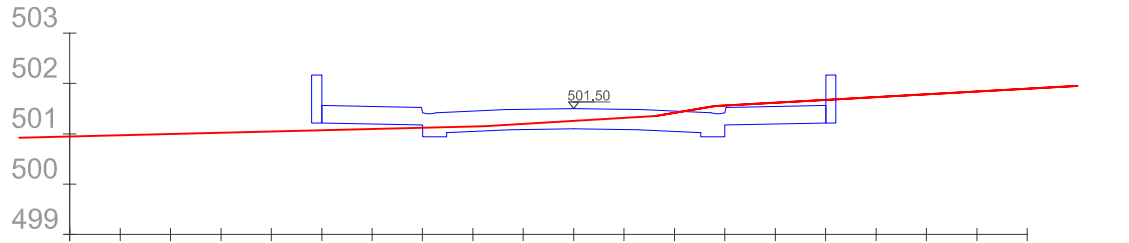
SECCION TRANSVERSAL 9
