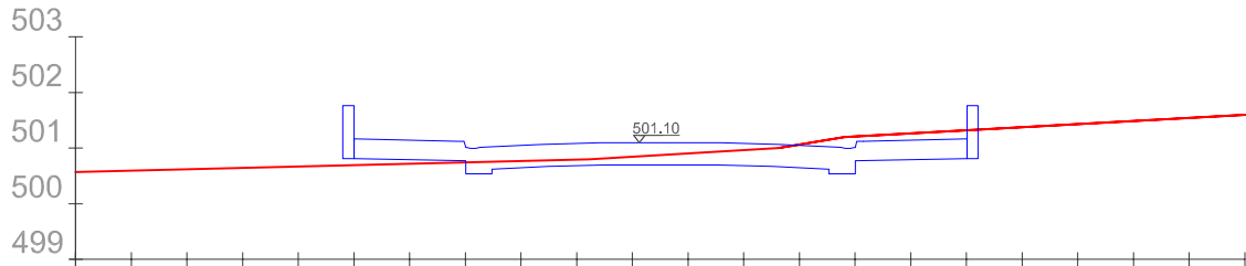
SECCION TRANSVERSAL 7
