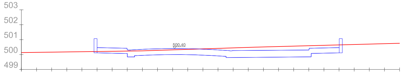
SECCION TRANSVERSAL 1
