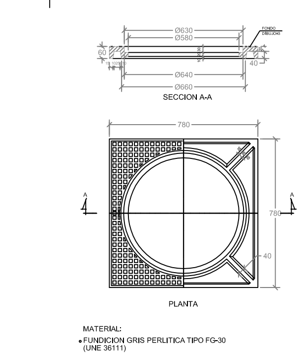
INSTALACION PLUVIALES
