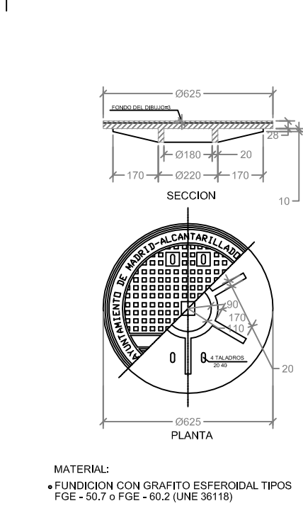
CERCO PARA POZO DE REGISTRO EN CALZADA
