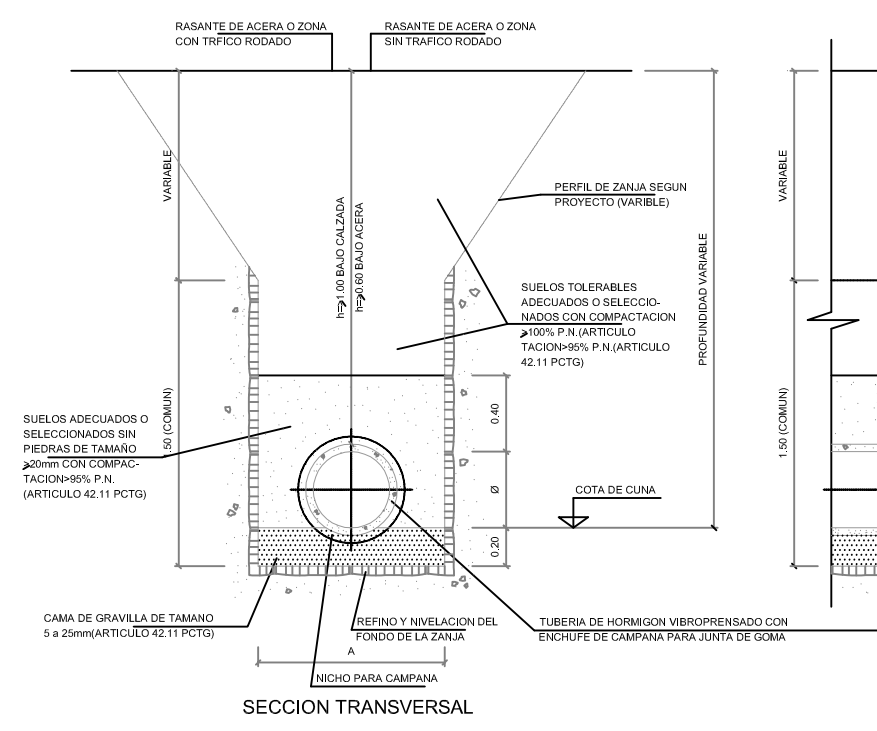
SECCION TIPO DE ZANJA PARA TUBULARES DE HORMIGON EN MASA (Ø 30 a 60 cm.) EN TERRENOS ESTABLES
