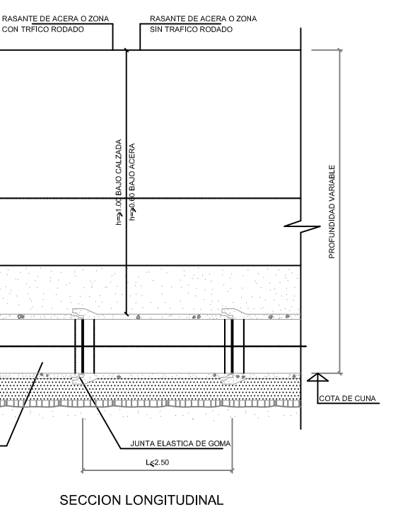
TAPA PARA POZO DE REGISTRO O ABSORBEDERO
